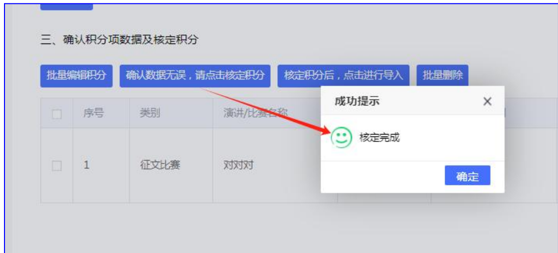
图 14 核定积分
